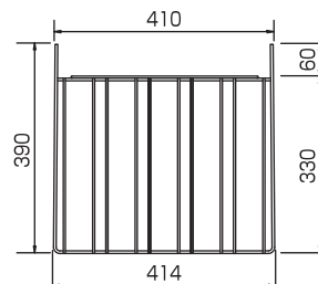
◆ワイヤー棚(最上棚)寸法図
