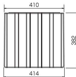
◆ワイヤー棚(下段棚)寸法図
