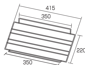
◆ワイヤー棚(下段棚)寸法図
